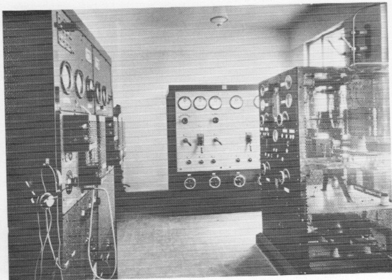
Interiør fra Bodø Kringkaster i 1932. Til venstre lavfrekvensenheten (Modulator). Til høyre høyfrekvensenheten. Høyfrekvenseffekten (programmet) føres ut gjennom vegg til antenner. Midt imot ses apparatet for fordeling av nettspenning til likerettere og roterende omformere. Foto: Helgesen.
